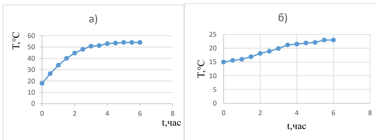
1-сурет. А) су температурасының 50 Гц кезіндегі қыздыру ұзақтығына тәуелділігі; б) үй-жай температурасының 50 Гц кезіндегі қыздыру ұзақтығына тәуелділігі
